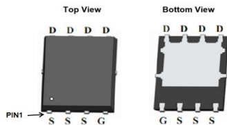
PDFN5X6-8L
