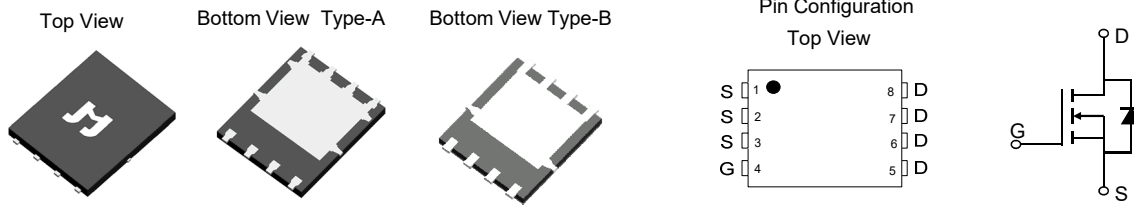
PDFN5x6-8L
